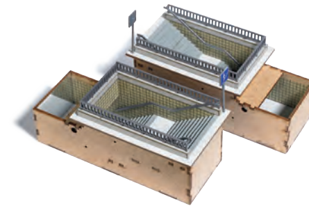
H0 1465 Fußgängerunterführungen € 37,99 Bausatz für 2 Fußgängerunterführungen. Größen jeweils: Straßenebene 87 x 53 mm. Treppenabgang 117 x 44 mm. Einbautiefe 40 mm.
